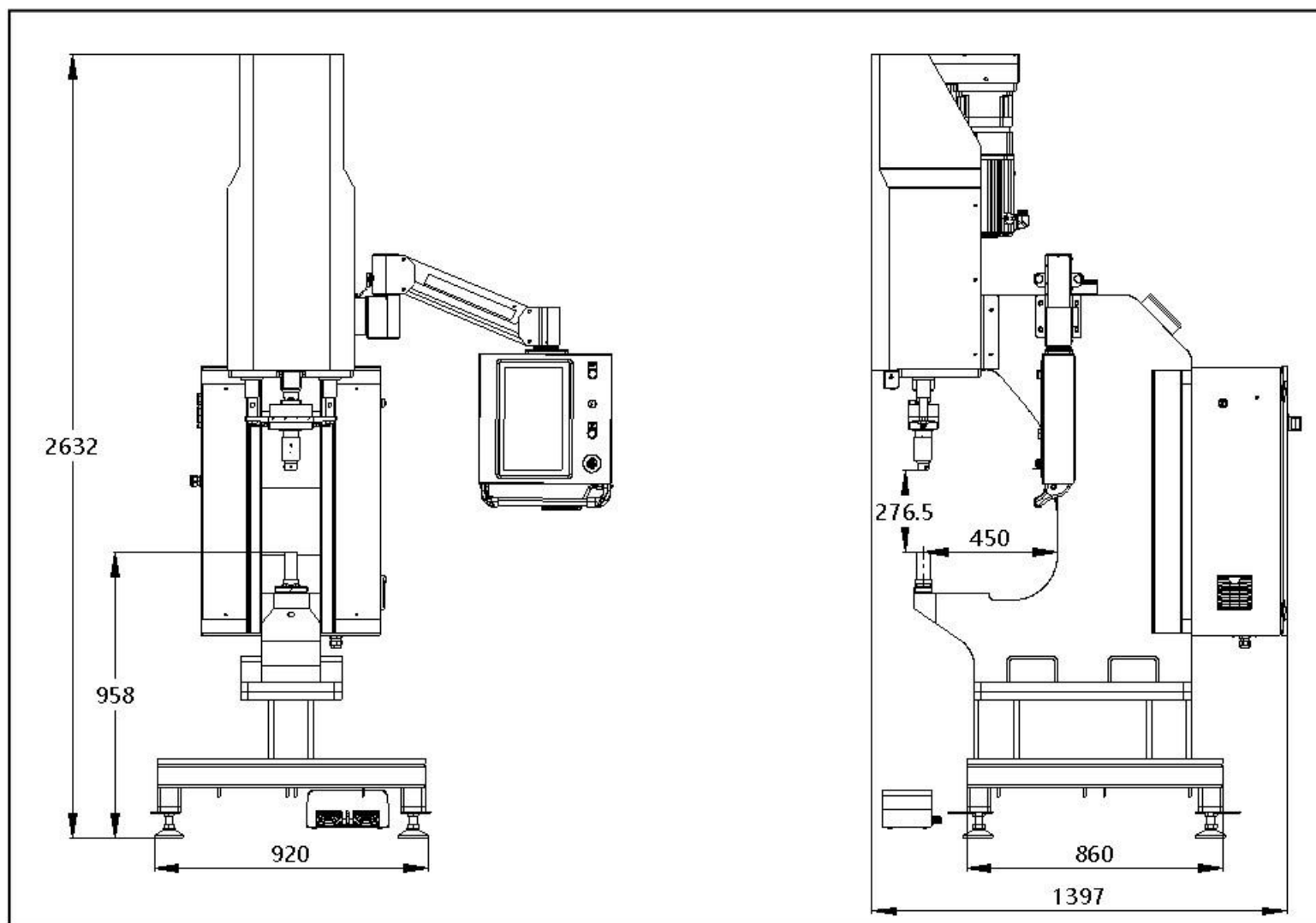
图 1-1 PA80 E-drive 伺服压机外形尺寸图
